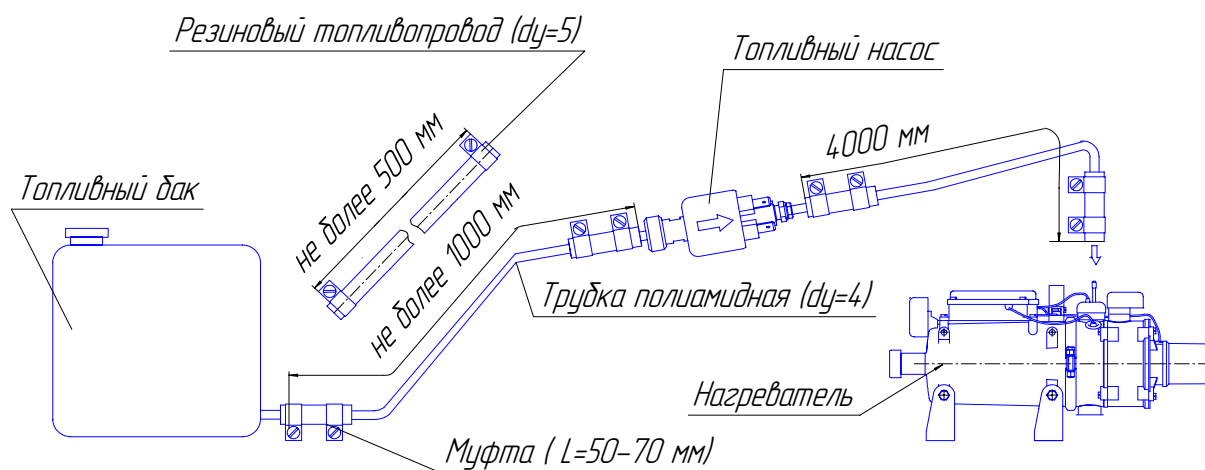
Рис. 7- Схема присоединения топливопровода к узлам подогревателя
