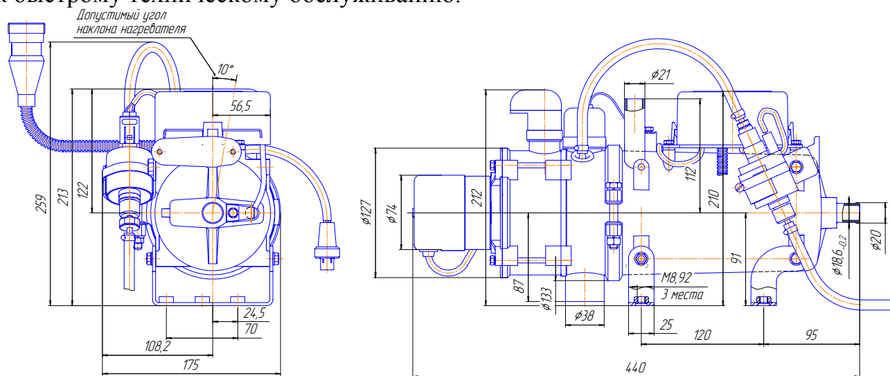
Рисунок 5- Допустимые рабочие положения нагревателя
